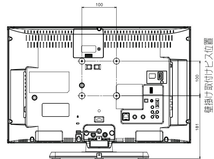
壁掛け取付けビス位置
