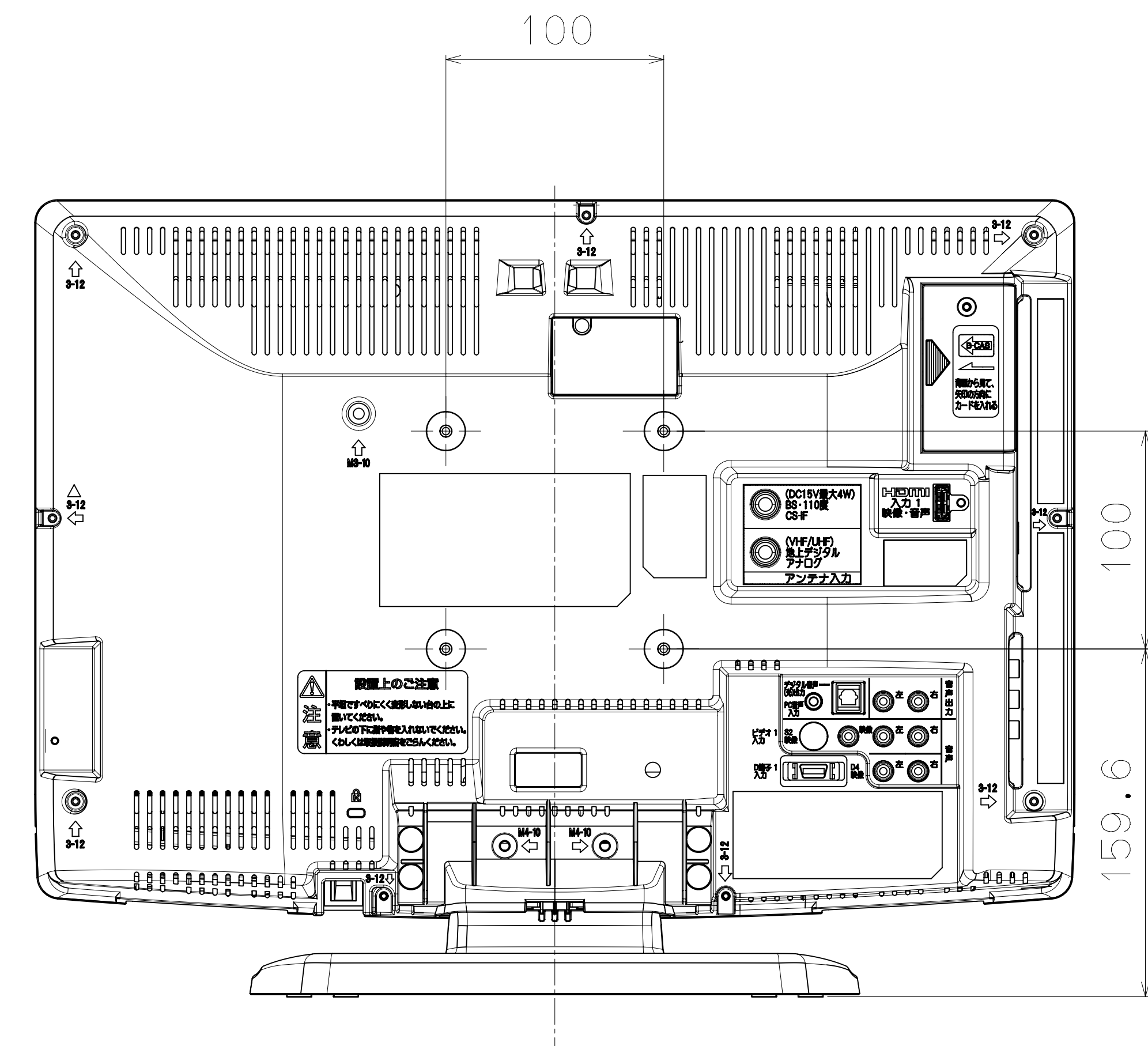
壁掛け取付ビス位置
