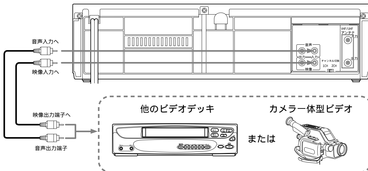
本機（背面）
