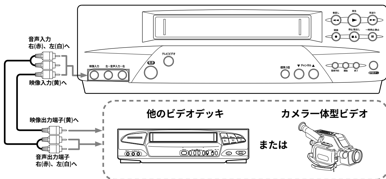
本機（前面）
