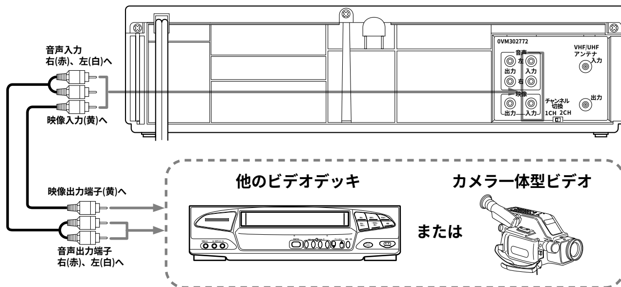
本機（背面）
