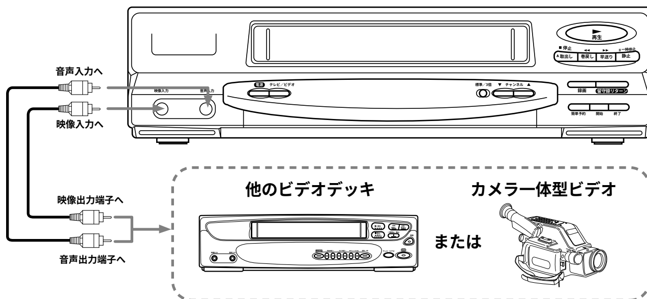
本機（前面）
