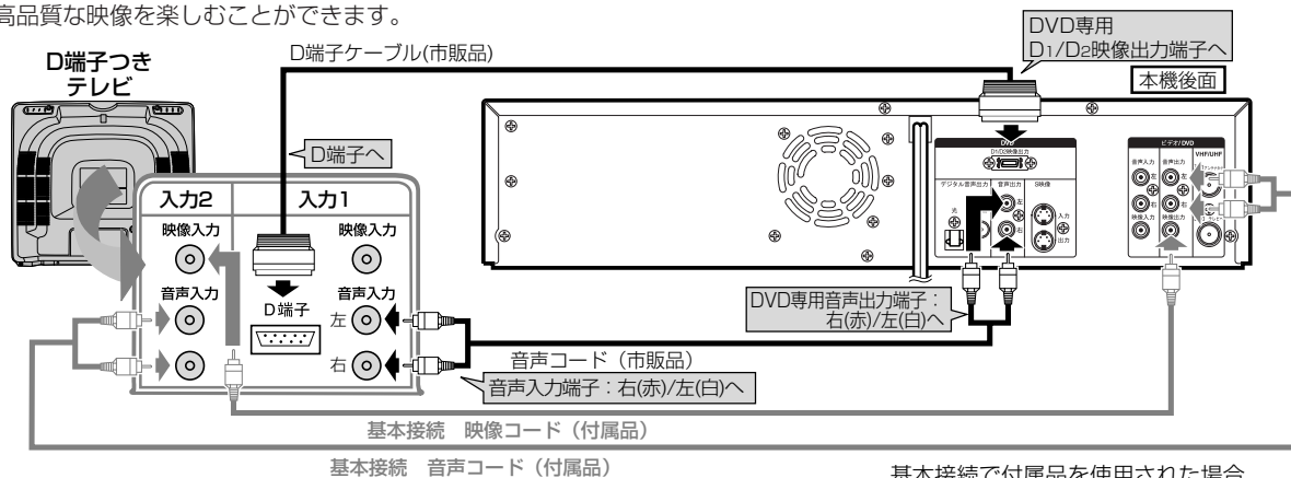
基本接続 音声コード(付属品)
