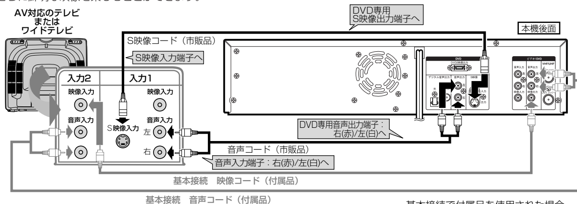
基本接続 音声コード(付属品)
