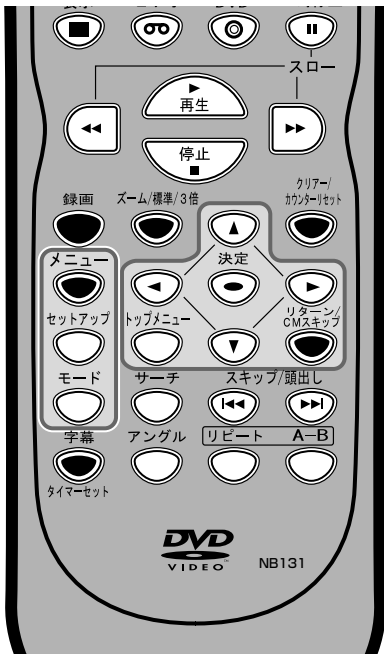
図2 リモコン 操作ボタン
